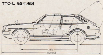
TTC-L GS寸法図
