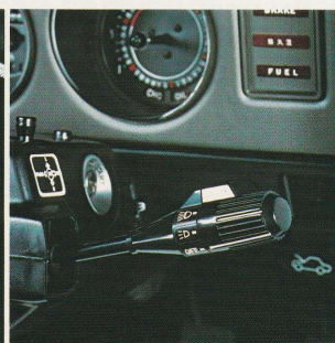
●ライトコントロールレバー ターニングナル、ライティング、デイマー、ヘッドランプホーンの各スイッチを集中一体化。全車に標準。
