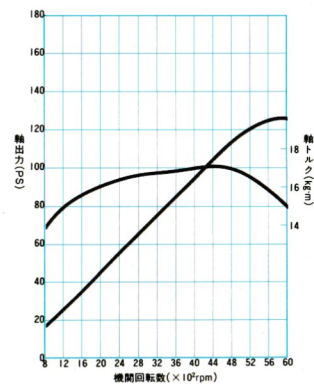
L20E ECCS エンジン性能曲線
