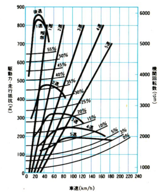
TURBO 2シーター走行性能曲線 OD付5速フロアシフト
