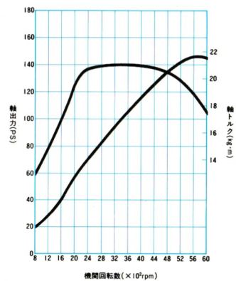
L20E・T ECCS TURBO エンジン性能曲線
