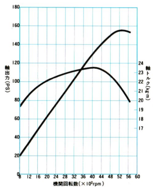
L28E G-ECCS エンジン性能曲線
