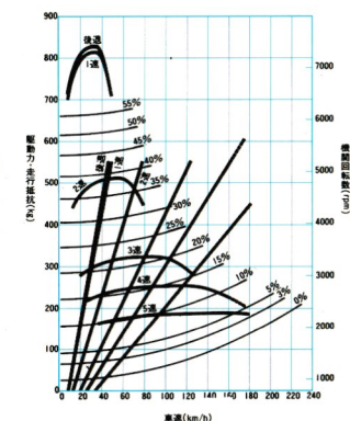
2800cc 2シーター走行性能曲線 OD付5速フロアシフト
