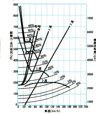
2000cc 2シーター走行性能曲線 ロックアップ付オートマチック
