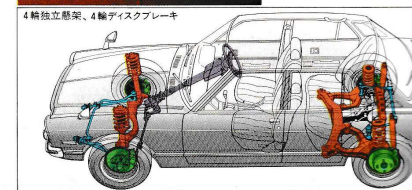
4輪独立懸架、4輪ディスクブレーキ
