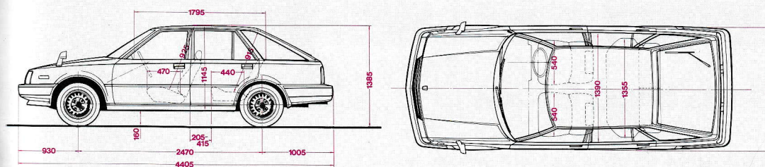
●5ドアハッチバック(1800ZX-E) 2面図
