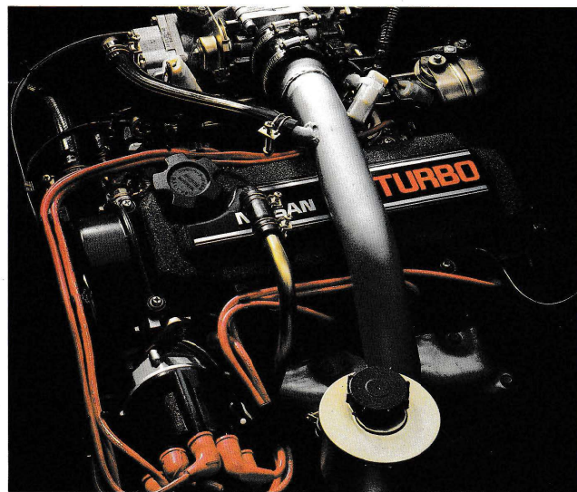
CA18E・T(ターボチャージャー付)型エンジン 軽量コンパクトな OHC・水冷・直列・4気筒 ニッサンが「新ガゼール」ではじめて世に送る新鋭ターボチャージャー付。 最高出力135ps/6000rpm、最大トルク20.0kgm/3600rpm。圧縮比は8.0。
