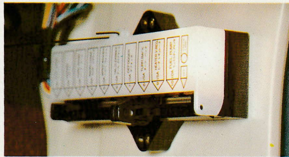
ヒューズチェッカー 電気系統のすべての点検はチェックノブをスライドさせるだけ。ひと目で具合の悪いところがわかります。
