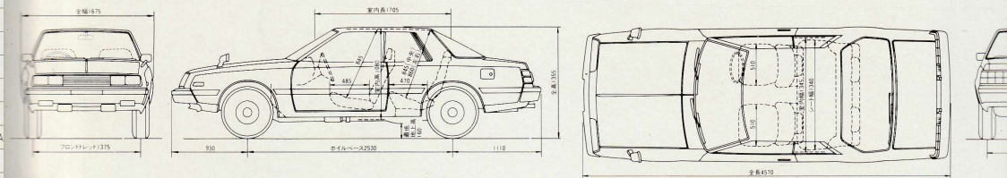
ギャランA四面図(2000GSR) 単位=mm
