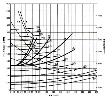
走行性能曲線図(2by2、3000ccニッサンマチック車)
