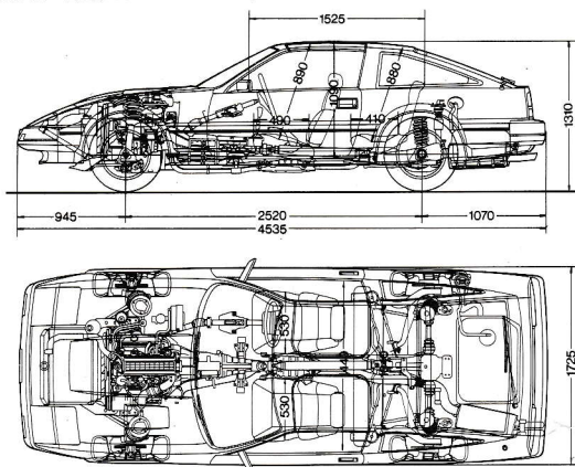
●2BY2二面図(300ZX T-BAR ROOF)
