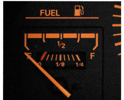
④ 親子メーター式燃料計
