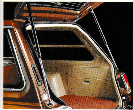
テールゲートストラット 圧縮ガス封入式ですので、いつもテールゲートの開閉は軽くスムーズです。
