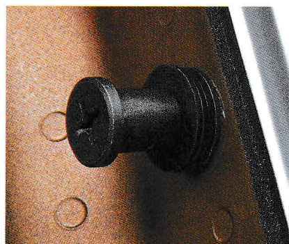
テールゲートロック 左右2ヶ所のサイドストライカ方式ですので、大切な商品を傷つけません。
