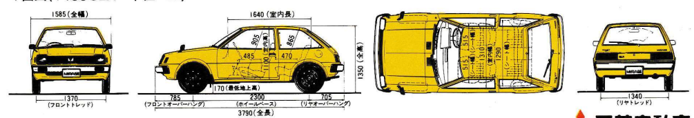
4面図(1400GLX・単位=mm)
